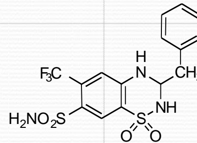
Bendroflumethiazide
