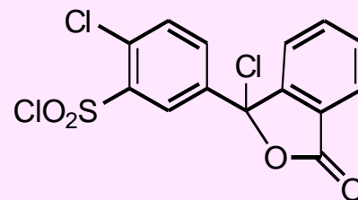
2-chloro-5-(1-chloro-3-oxo-1,3-dihydroisobenzofuran-1-yl)benzene-1-sulfonylchloride
