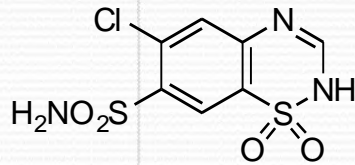
Chlorothiazide
