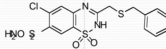
Benzthiazides
