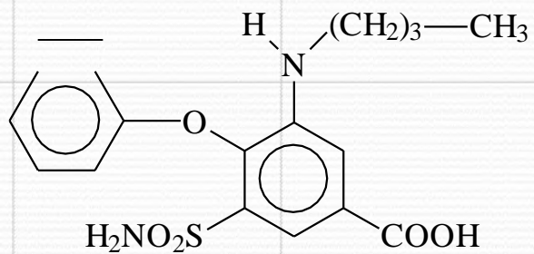
Bumetanide (Bumex)
