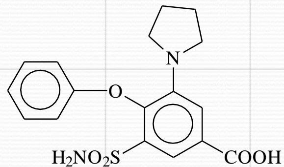
Piretanide
