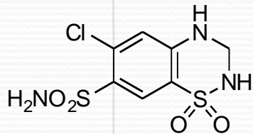
Hydrochlorothiazide
