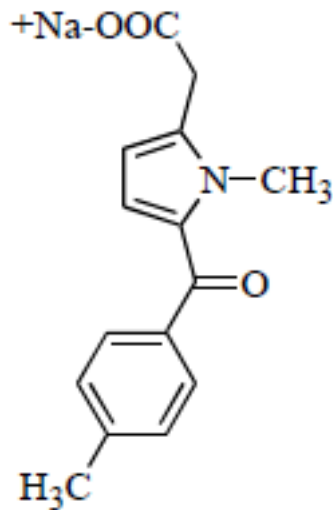
Tolmetin
