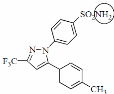
Celecoxib, Celebrix®
